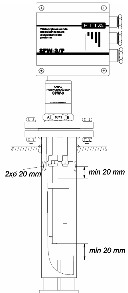
Przykład montażu sondy w płaszczach kotłów lub zbiorników
